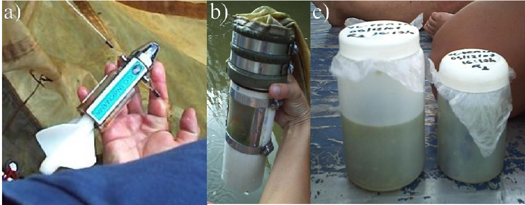
FIGURA 5 - (a) Fluxômetro, (b) copo coletor da rede e (c) potes de polietileno utilizados nas amostragens.
